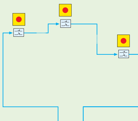
Principio paros de emergencia
