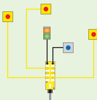
Instalación paros de emergencia con distribución Safety
